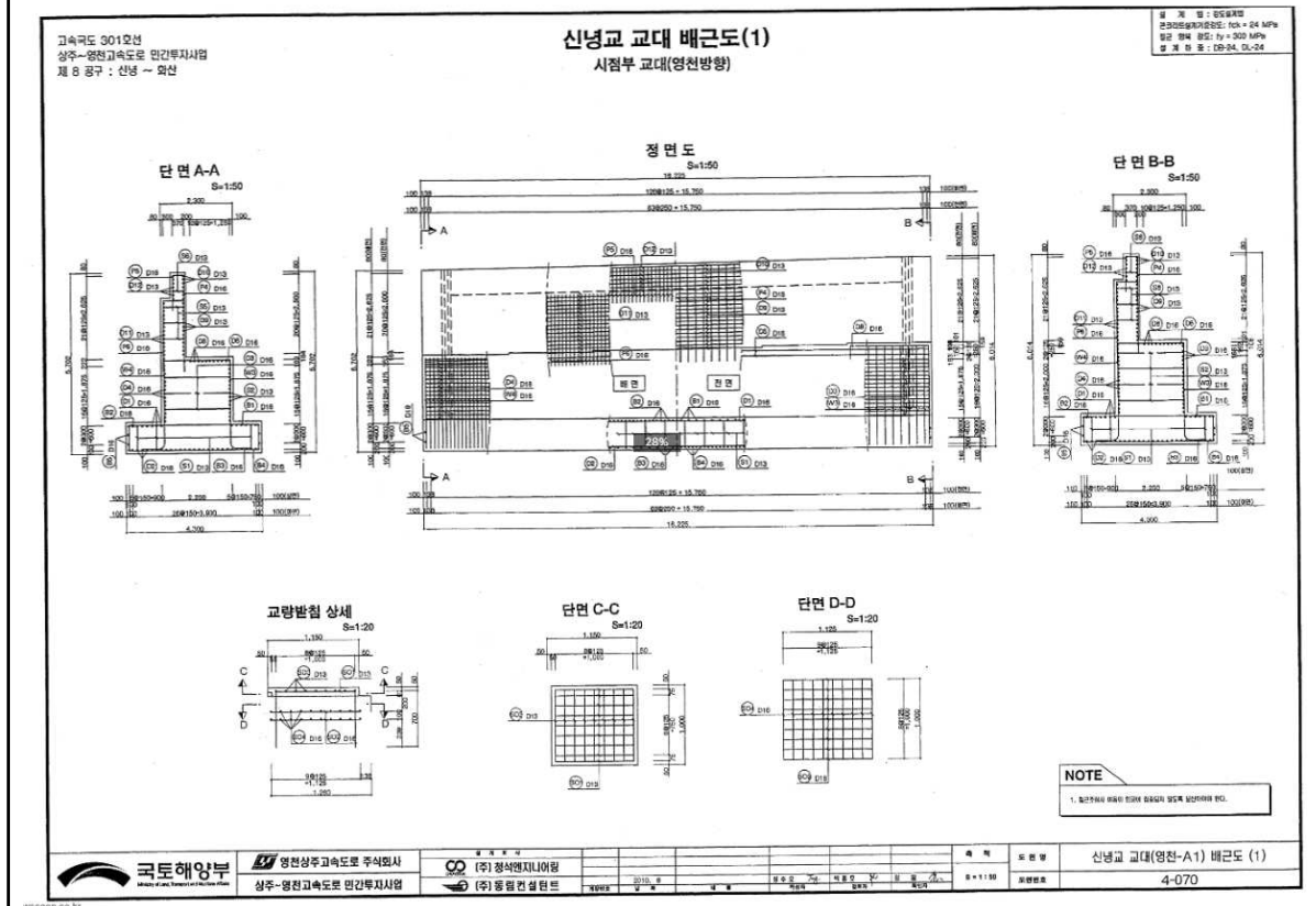
【그림 20.1.12】 교대 배근도
